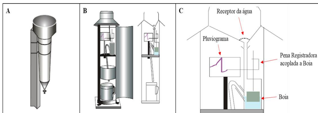
FIGURA 2 – Esquema de um Pluviômetro Ville de Paris (A) e de um Pluviógrafo de boia (B) e detalhamento do método de acumulação de água e registro da precipitação do Pluviógrafo.
