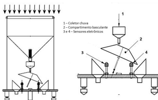
FIGURA 3 - Esquema de pluviógrafo de báscula.
