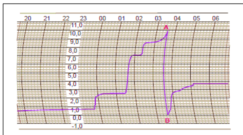
FIGURA 4 – Parte de um pluviograma. A escala horizontal representa as horas do dia e a escala vertical a lâmina precipitada em mm.
