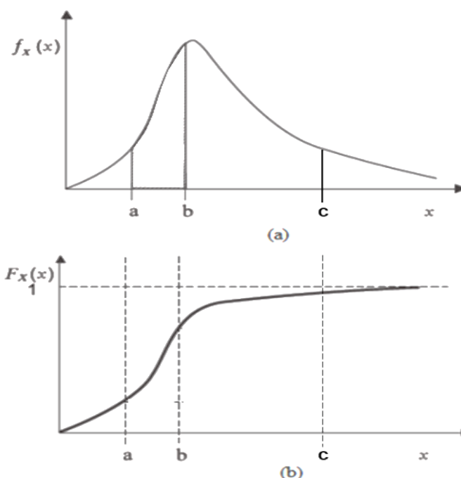
FIGURA 5 - Funções densidade e acumulada de probabilidades de uma variável contínua.
