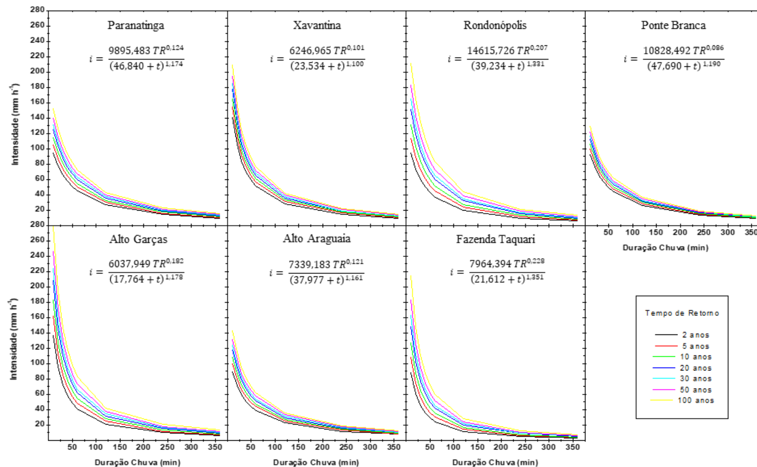
FIGURA 8 - Curvas de Intensidade de precipitação máxima para diferentes períodos de retorno, ajustados por meio das equações IDF para os postos pluviográficos do bioma Cerrado, no Estado de Mato Grosso.
