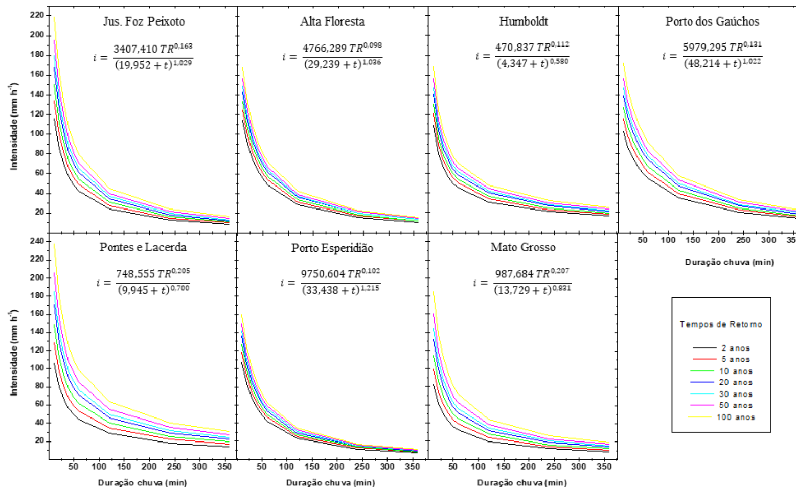
FIGURA 7 - Curvas de Intensidade de precipitação máxima para diferentes períodos de retorno, ajustados por meio das equações IDF para os postos pluviográficos dos biomas Amazônia e Ecótono dos Biomas Cerrado-Amazônia-Pantanal, no Estado de Mato Grosso.
